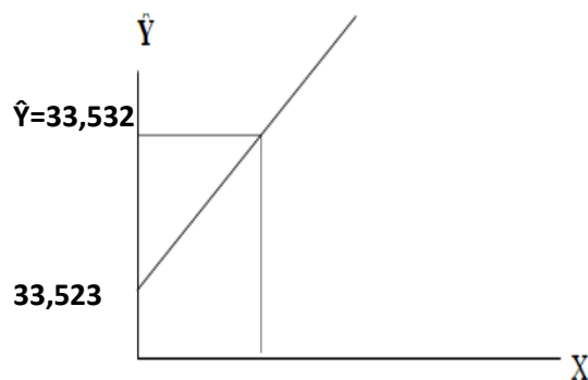
Gambar Persamaan Garis Regresi X terhadap Y
